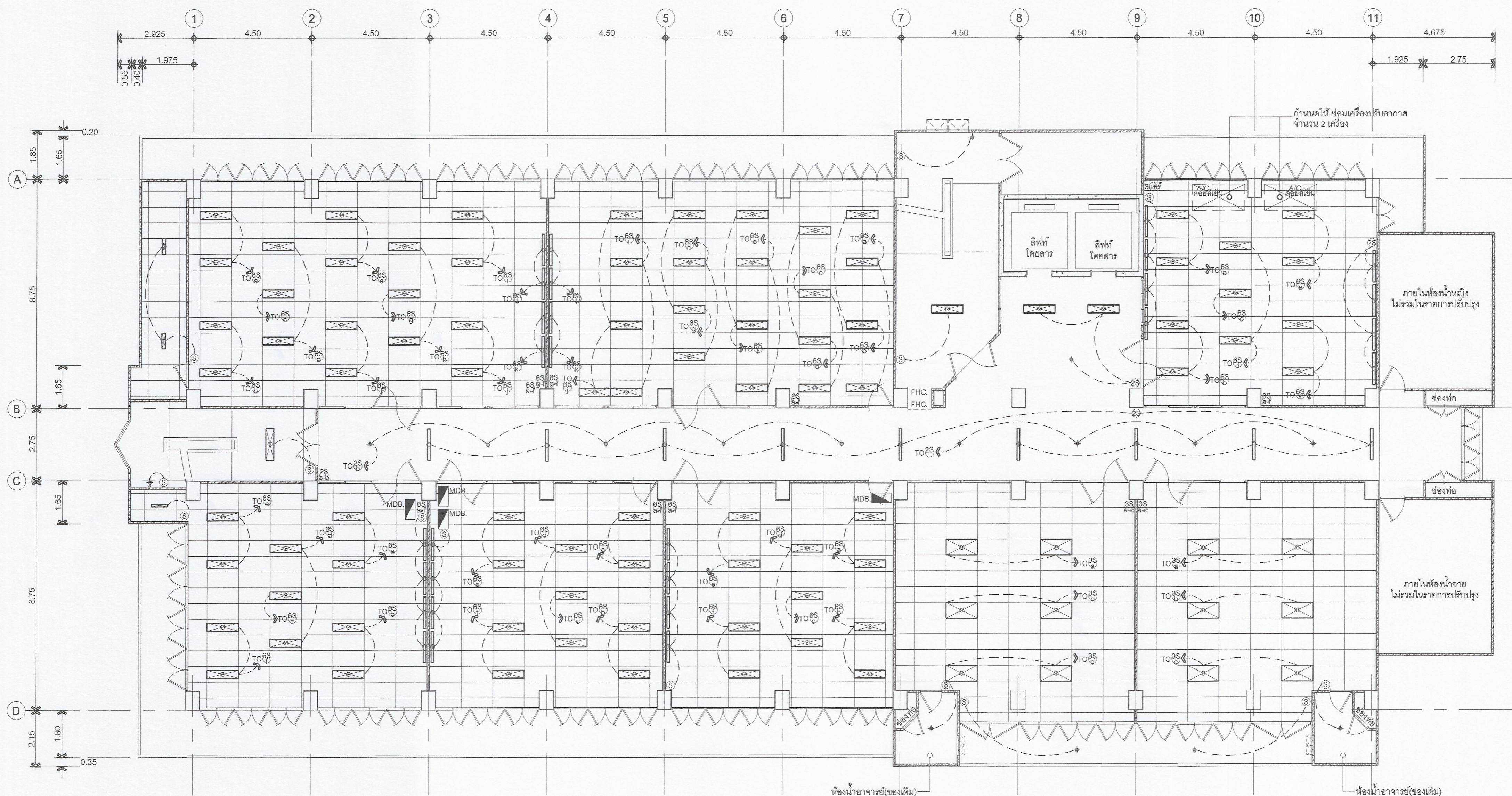
10th. FLOOR PLAN ไฟฟ้าแสงสว่าง ก่อนปรับปรุง มาตราส่วน 1 : 100
