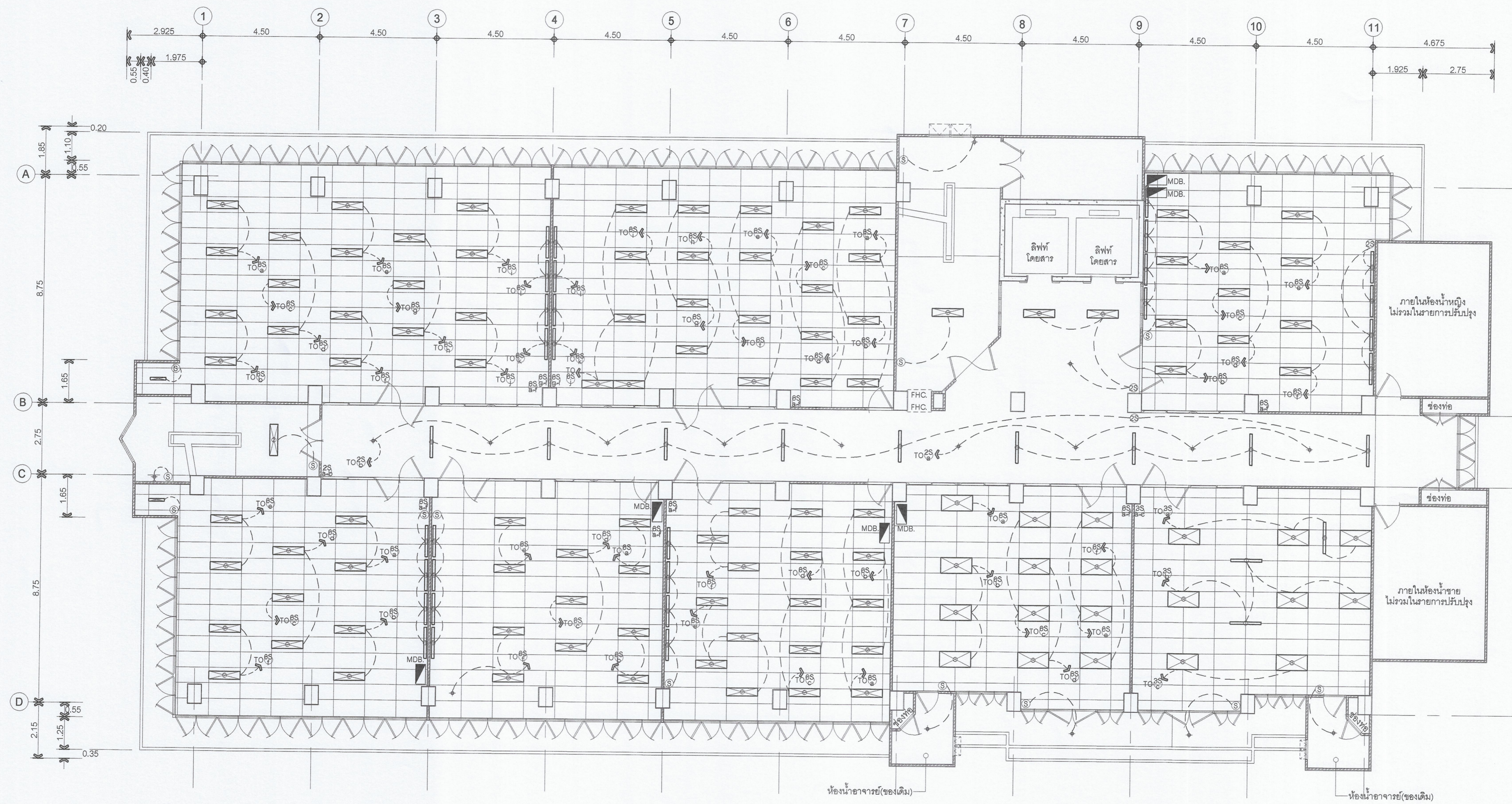
9th. FLOOR PLAN ไฟฟ้าแสงสว่าง ก่อนปรับปรุง มาตราส่วน 1 : 100
