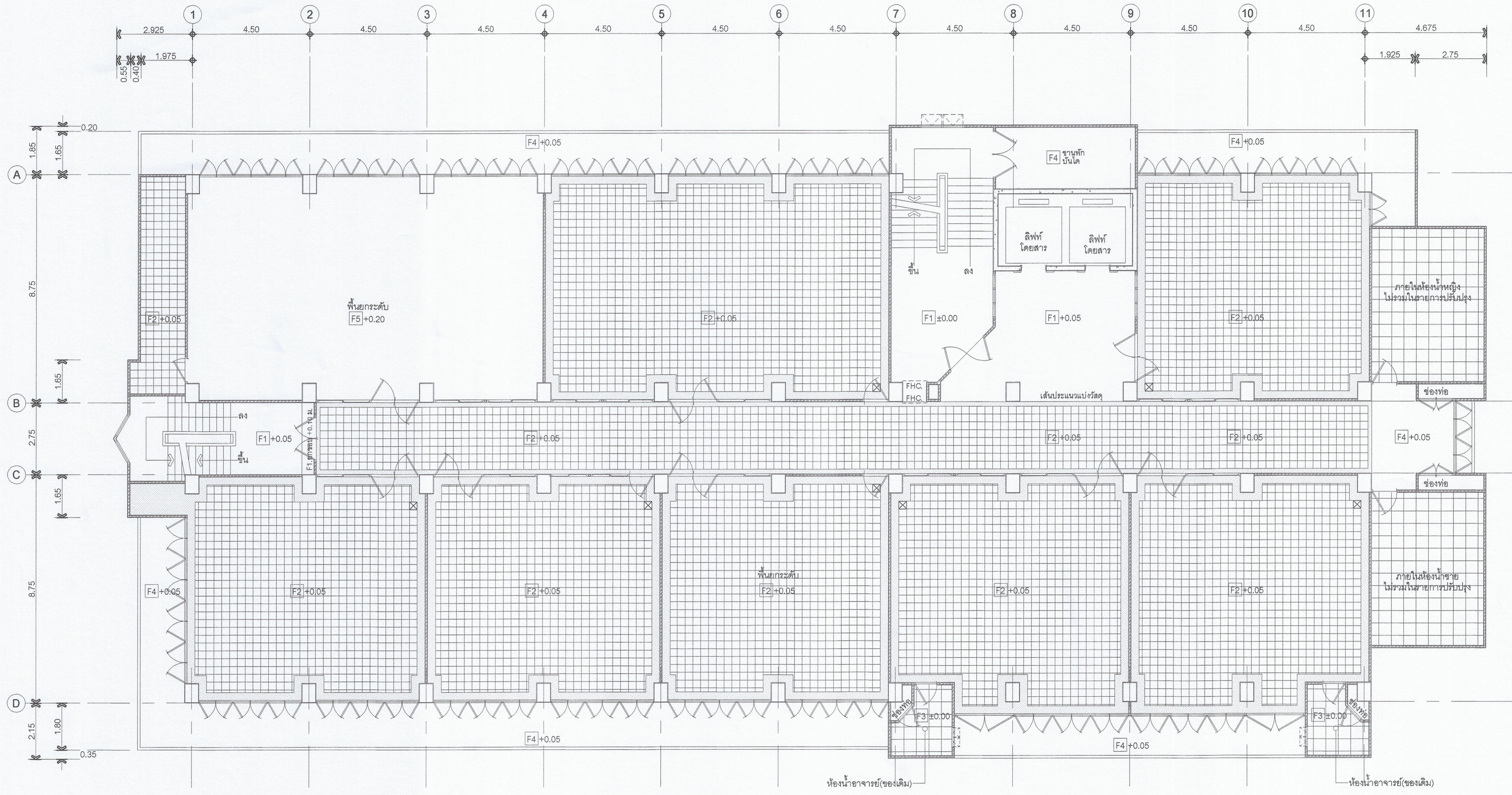
10th. FLOOR PATTERN PLAN ก่อนปรับปรุง มาตราส่วน 1 : 100
