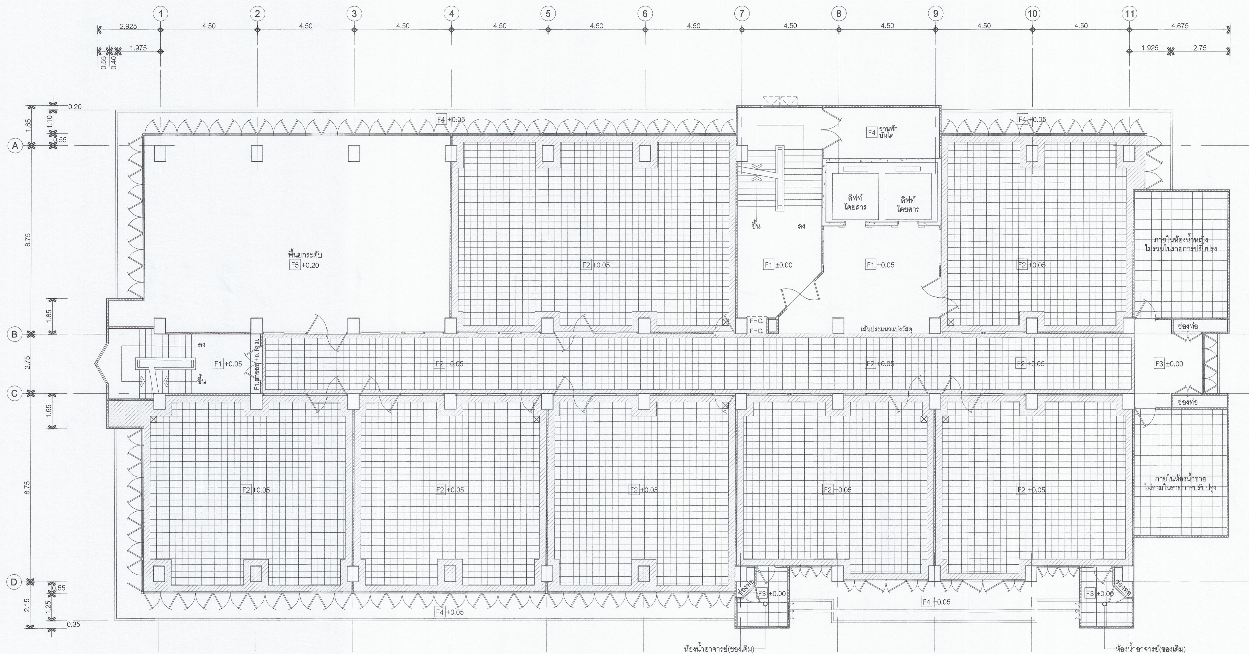
9th. FLOOR PATTERN PLAN ก่อนปรับปรุง มาตราส่วน 1 : 100
